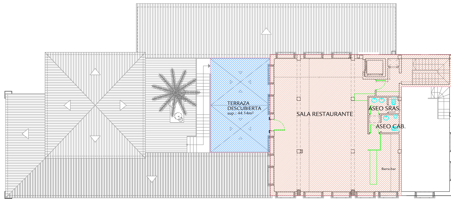
PLANTA PRIMERA
