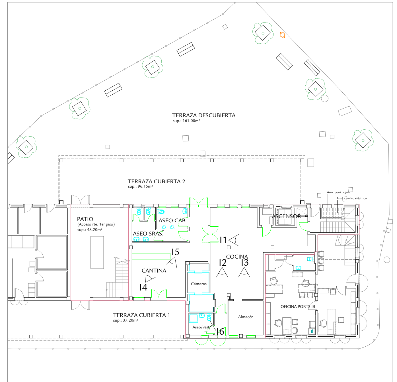
PLANTA BAJA. E:1/200
