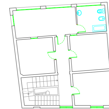
PLANTA PISO 1
