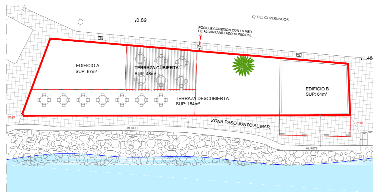
PROPUESTA ESTADO FUTURO E:1/300
