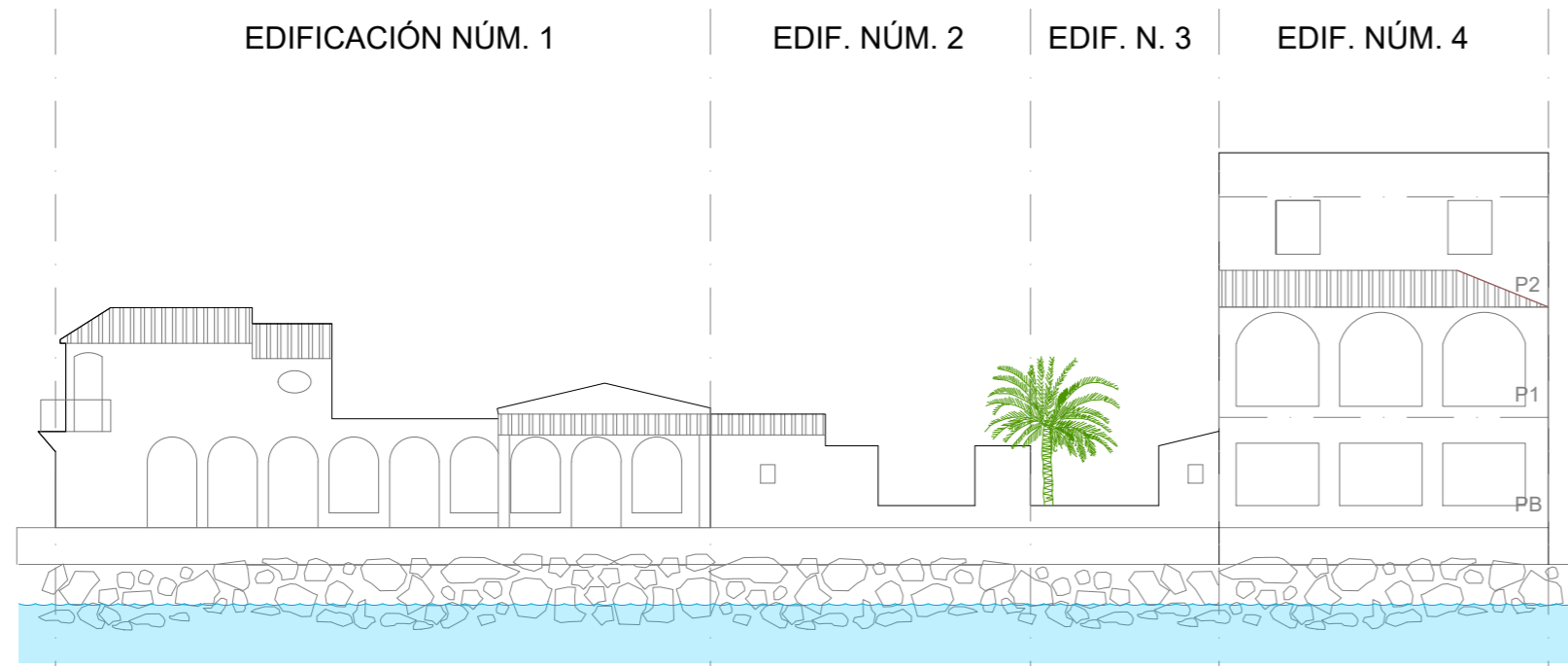
ALZADO ACTUAL (VISTA DESDE EL MAR) E:1/200
