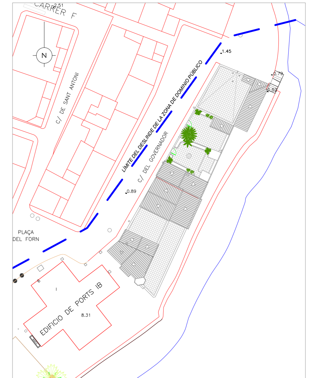
SITUACIÓN Y PLANTA CUBIERTA E:1/400
