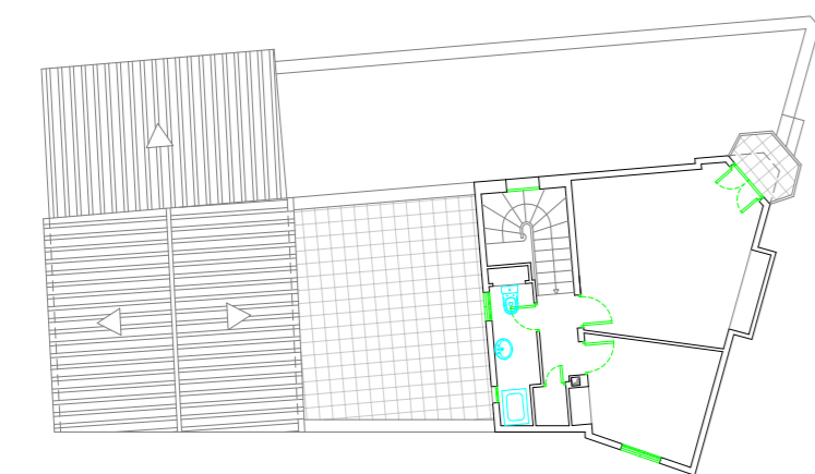
PLANTA PISO
